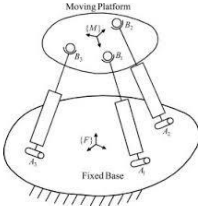
Паралелен робот Parallel robot
